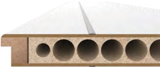
Schnitt Metaopt, Standardeinlage RSP
