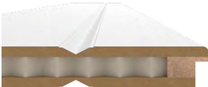
Schnitt Country, Standardeinlage Wabe
