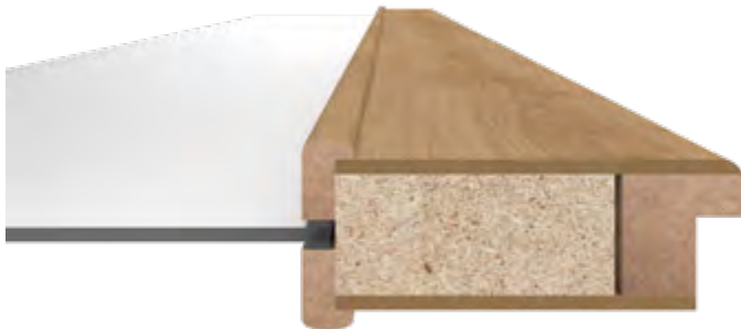
Glasleiste Nr. 14
