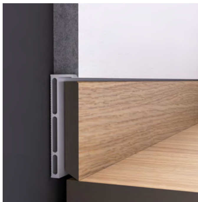
Profil C70 in Massivbauwand
